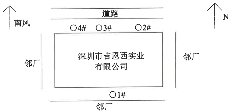
附图：无组织废气采样点位示意图
